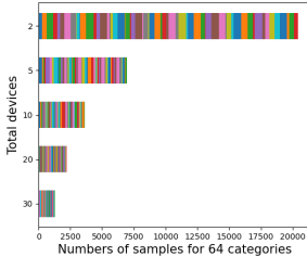
Fig. 7: Non-IID data.
